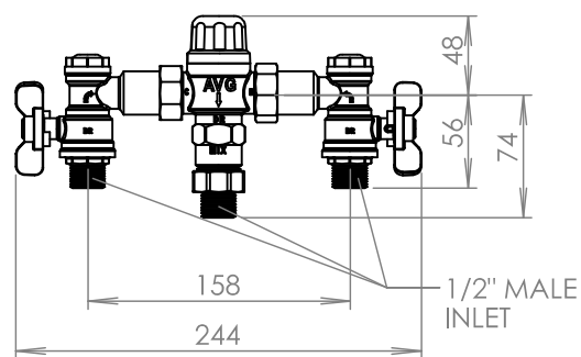
TMV DIMENSIONS
